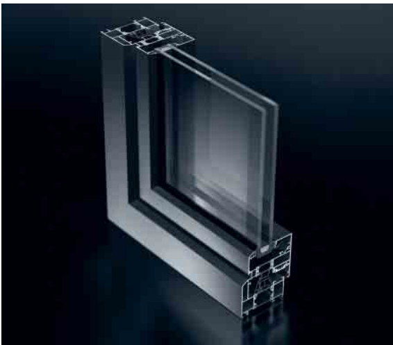
Schüco Fenster AWS 65 RL System mit abgeschrägter Außenkontur Schüco window AWS 65 RL System with bevelled exterior contour
